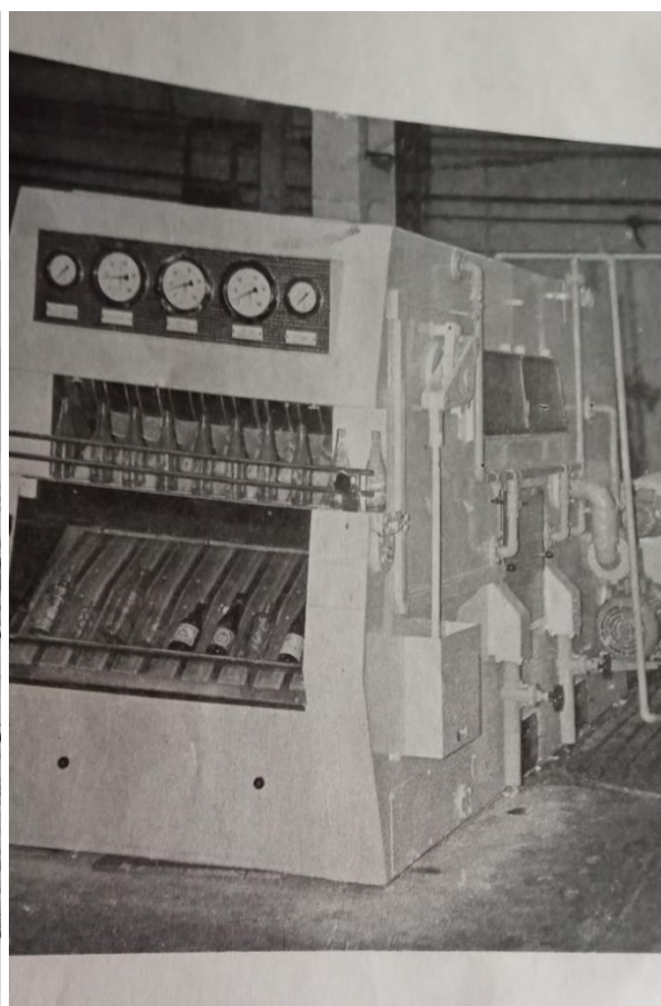
Myjka LMB - 25
